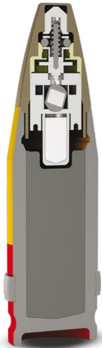
Projétil com espoleta de ogiva
